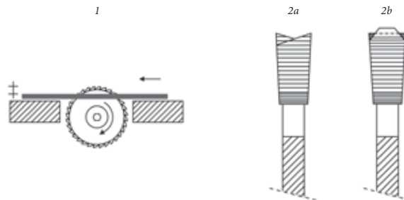
fig 8. 1. Instelhoogte – 2a. Wisseltand – 2b. Trapezium-vlaktand
